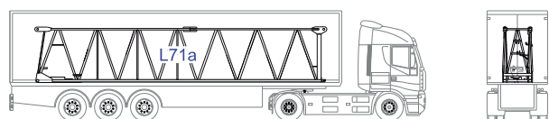
CL7-RI10-RS10-C1
