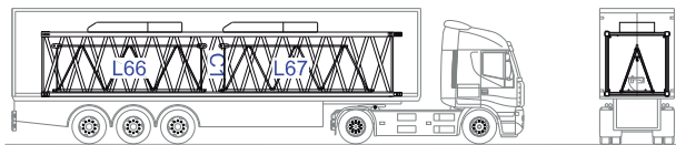
C1-L66-L67-2xCP2
