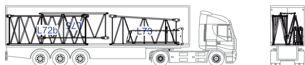
L72a-L72b-L73a-L75-2xC1
