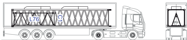
C1-L76-2xCP2
